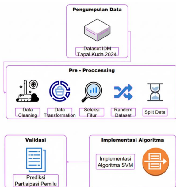
Gambar 1. Tahapan Penelitian
