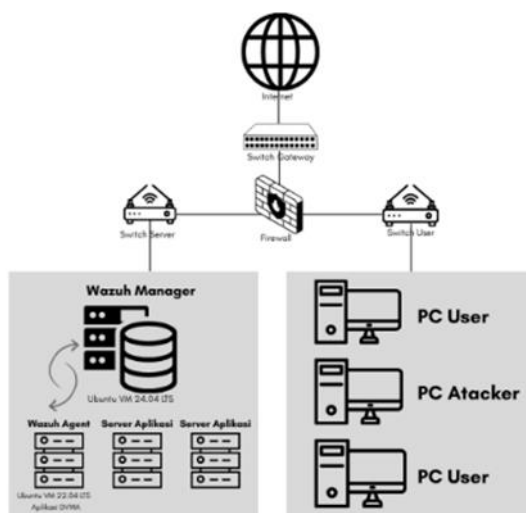
Gambar 2. Topologi Pengujian
